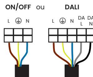
Schéma de câblage DALI
