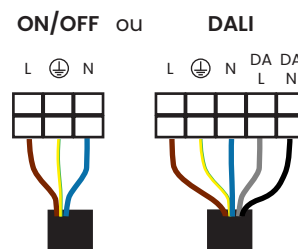
Schéma de câblage DALI
