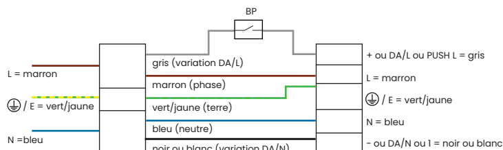
Schéma de câblage DALI
