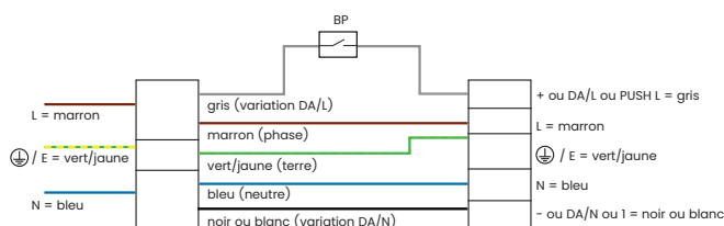
Schéma de câblage DALI
