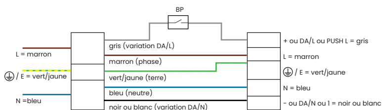
Schéma de câblage DALI
